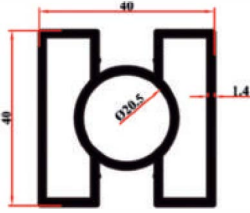
KRM 9125 1 40x40 Çift Kanallı 0,890 Kg/Mt
