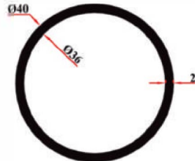
KRM 9106 40x2 mm Boru 0,64 Kg/Mt
