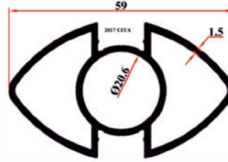
KRM 9131 1 Badem Profil 0,874 Kg/Mt
