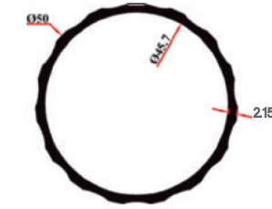
KRM 9105 50'lik Tırtırlı Boru 0,730 Kg/Mt
