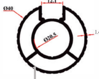
KRM 9111 40'lik Tek Kanallı Tırtırlı 0,801 Kg/Mt
