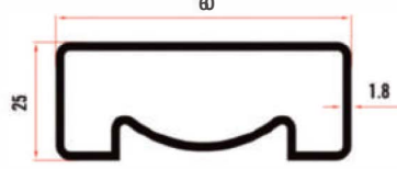
KRM 9123160x25 1 Kutu Profil 0,845 Kg/Mt
