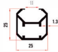
KRM 9127 1 25x25 Profil 0,460 Kg/Mt
