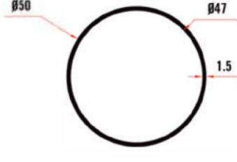
KRM 9103 50x1,5 mm Profil 0,625 Kg/Mt
