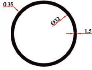
KRM 9114 35x1,5 mm Boru 0,426 Kg/Mt
