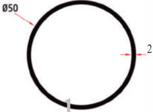
KRM 9101 50x2 mm Profil 0,817 Kg/Mt
