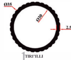
KRM 9115 35x2,5 mm Tırtırlı Boru 0,637 Kg/Mt
