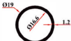
KRM 9117 19x1,2 mm Boru 0,181 Kg/Mt
