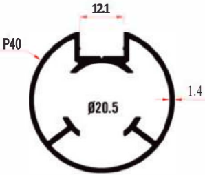
KRM 9109 40'lik Tek Kanallı 0,670 Kg/Mt
