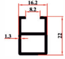
KRM 9128 1 Cam Kızağı 0,267 Kg/Mt
