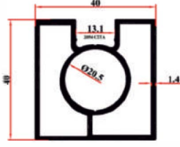
KRM 9126 1 40x40 Tek Kanallı 0,891 Kg/Mt
