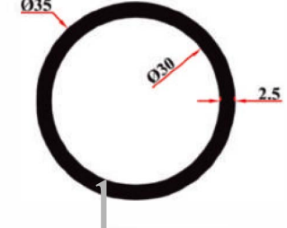
KRM 9111 35x2,5 mm Boru 0,691 Kg/Mt
