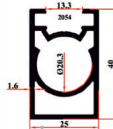
KRM 9135 1 40x25 Tek Kanallı 0,114 Kg/Mt
