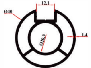
KRM 9108 40'lik Tek Kanallı 0,830 Kg/Mt
