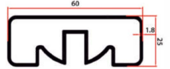
KRM 9124 1 60x25 Ortadan Kanallı 0,865 Kg/Mt
