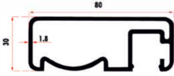
KRM 9121 1 80x30 Küpeşte Profil 1,240 Kg/Mt
