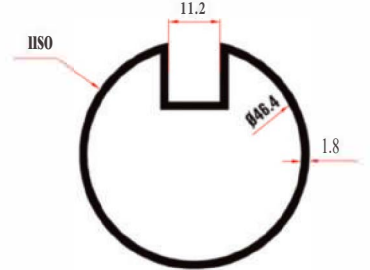
KRM 9104 50x1,8 Tek Kanallı Üst Kopeşte 0,900 Kg/Mt
