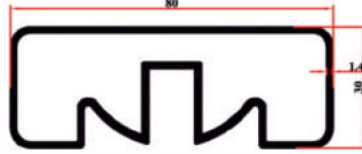
KRM 91221 1 80x30 Ortadan Kanallı 1,147 Kg/Mt
